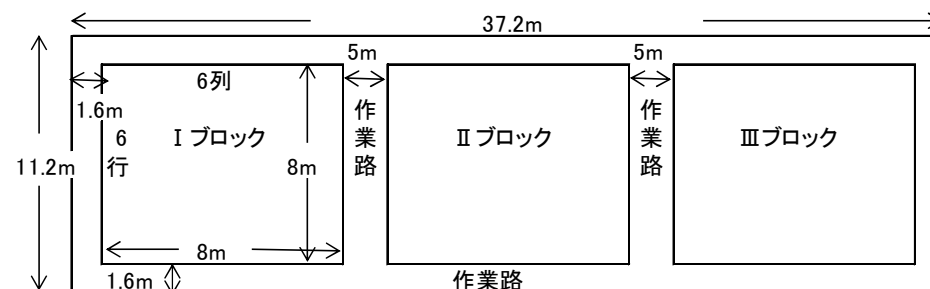
○スギミニチュア採種園全体の設計図 (2種類の特定期母樹により採種園を造成する場合)
