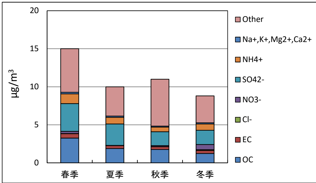
図3. 令和元年度 PM2.5季節別平均成分濃度
