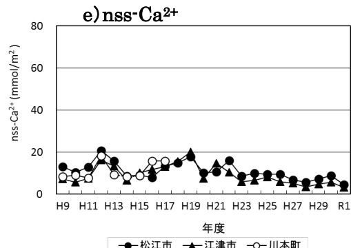
図4 県内3地点における主要イオン成分年別沈着量の経年変化(平成9~令和元年度)
