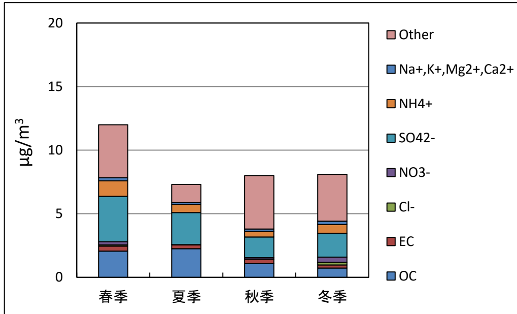
図1. 令和元年度 PM2.5季節別平均成分濃度
