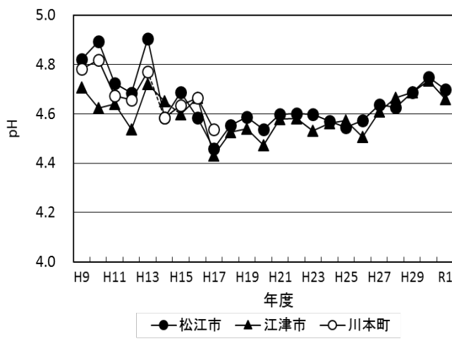
図2 年平均 pH の経年変化
