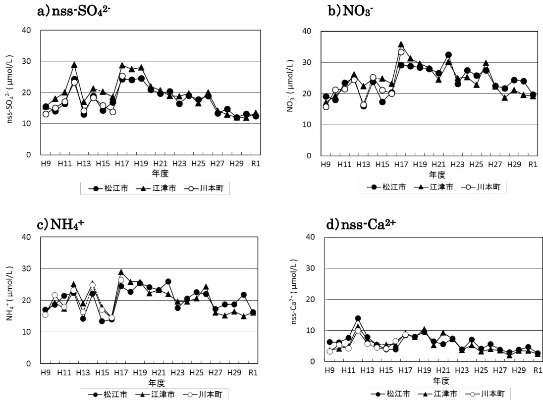
図3 県内3地点における主要イオン成分年加重平均濃度の経年変化 (平成9~令和元年度)
