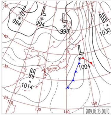
図1 2019年5月23日9時における日本域地上天気図
