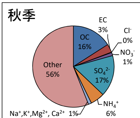
図4. 令和元年度 PM2.5季節別平均成分割合
