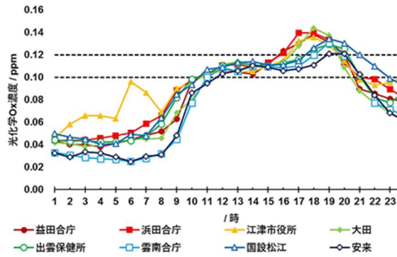
図3 2019年5月23日における光化学Ox濃度経時変化
