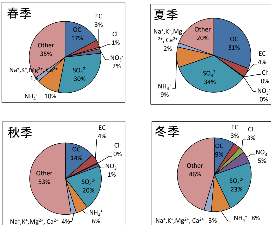
図2. 令和元年度 PM2.5季節別平均成分割合
