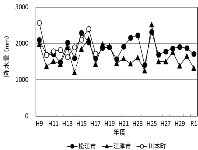
図1 降水量の経年変化
