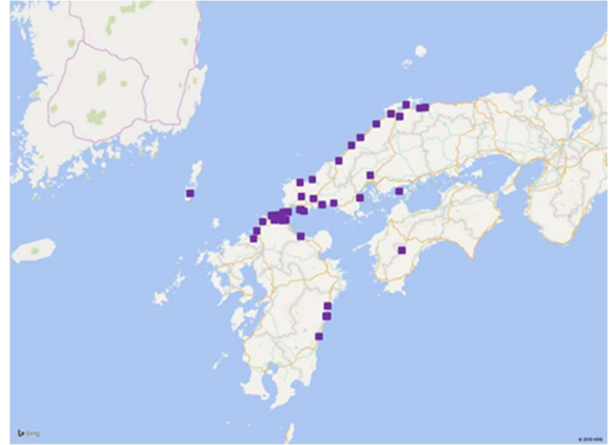
図4 2019年5月23日に中国・四国・九州地方で0.12 ppm以上の光化学Oxが観測された地点
