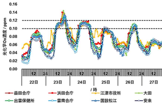
図2 2019年5月22日～27日における光化学Ox濃度経時変化
