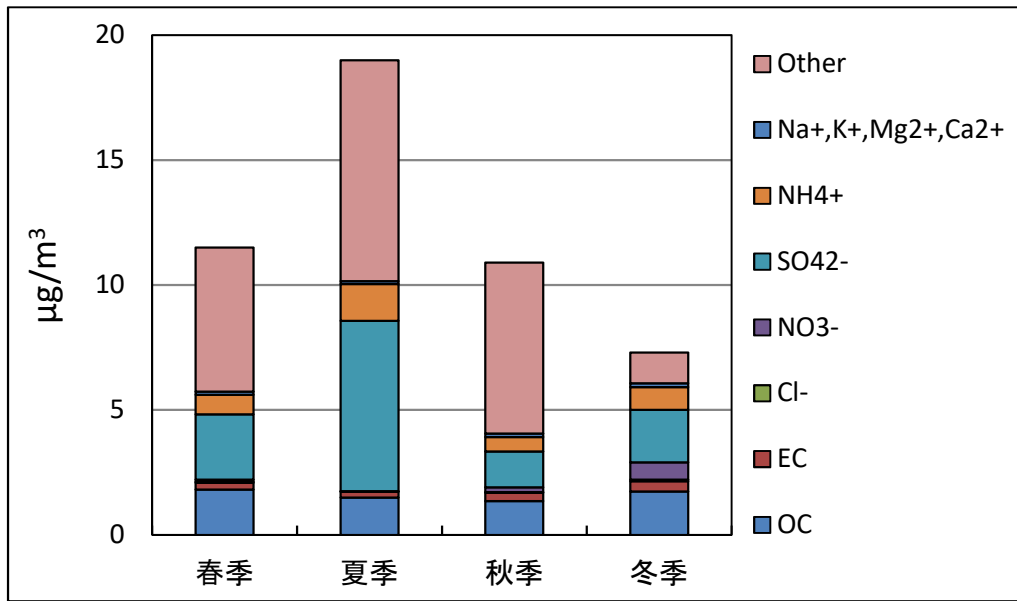
図3. 令和2年度 PM2.5季節別平均成分濃度
