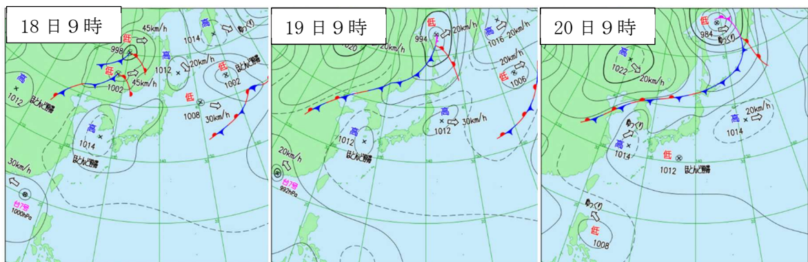
図 1 2020年8月18日から20日における天気図（気象庁HPより）
