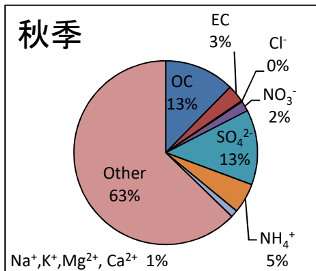
図4. 令和2年度 PM2.5季節別平均成分割合
