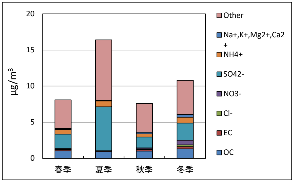
図1. 令和2年度 PM2.5季節別平均成分濃度
