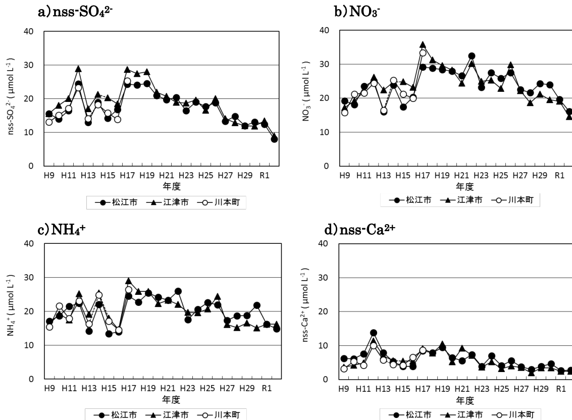
図3 県内3地点における主要イオン成分年加重平均濃度の経年変化(平成9~令和2年度)
