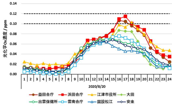
図2 2020年8月20日の県内8局における光化学O x 濃度の経時変化
