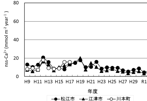
図 4 県内 3 地点における主要イオン成分年別沈着量の経年変化 (平成 9~令和 2 年度)
