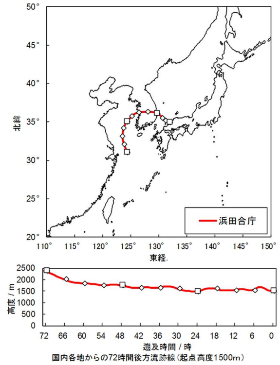
図3 2020年8月20日17時の浜田合庁における後方流跡線解析結果
