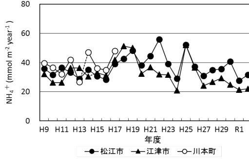
図 4 県内 3 地点における主要イオン成分年別沈着量の経年変化 (平成 9~令和 2 年度)
