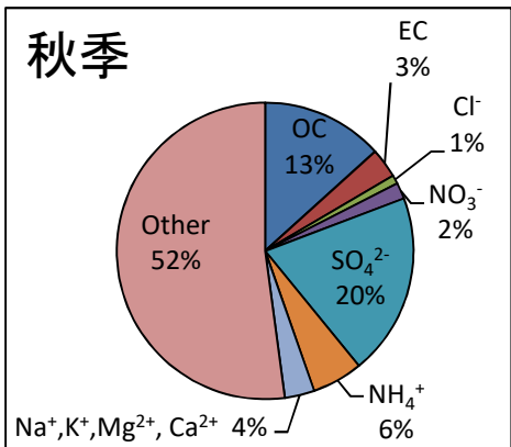
図2. 令和2年度 PM2.5季節別平均成分割合
