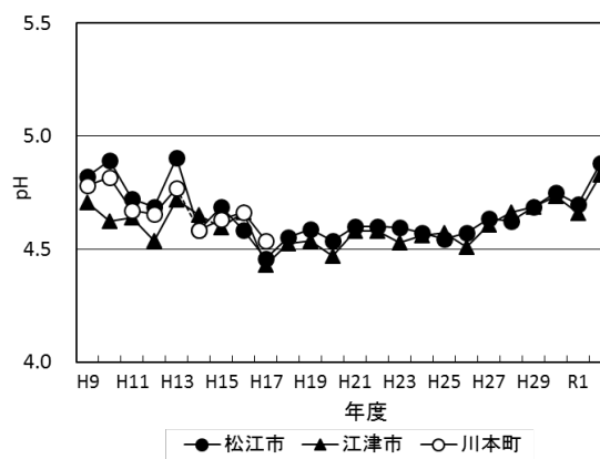
図2 年平均 pH の経年変化
