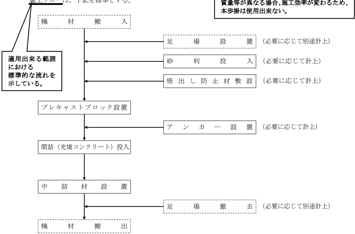
図1.1 施工フロー
