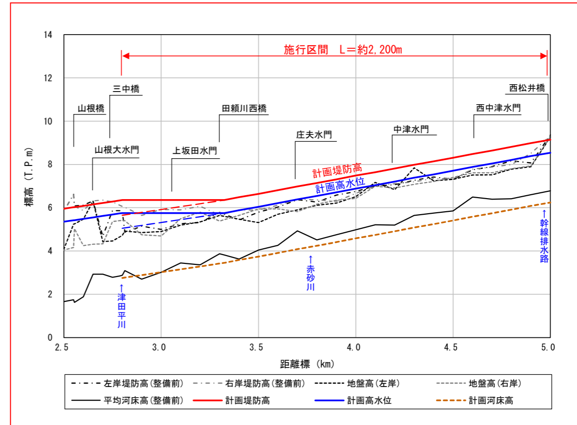
図 4.1-12 田頼川縦断面図
