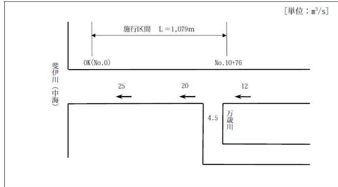
図-3.1.2(12) 木戸川整備計画目標流量図
