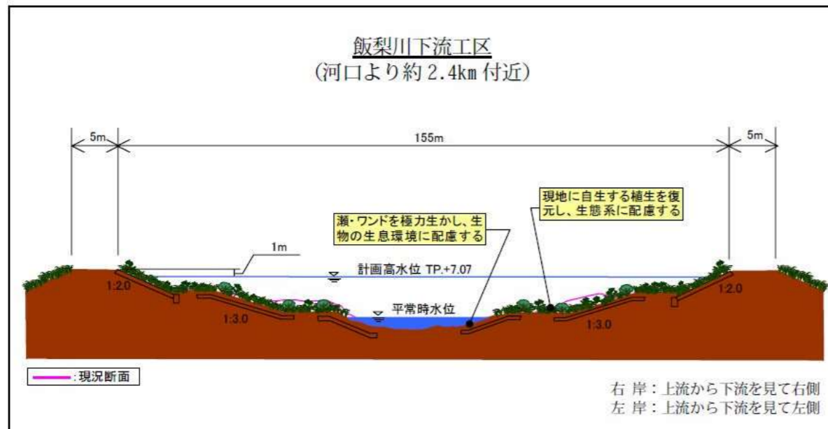
図-3.1.2(4) 標準横断面図
