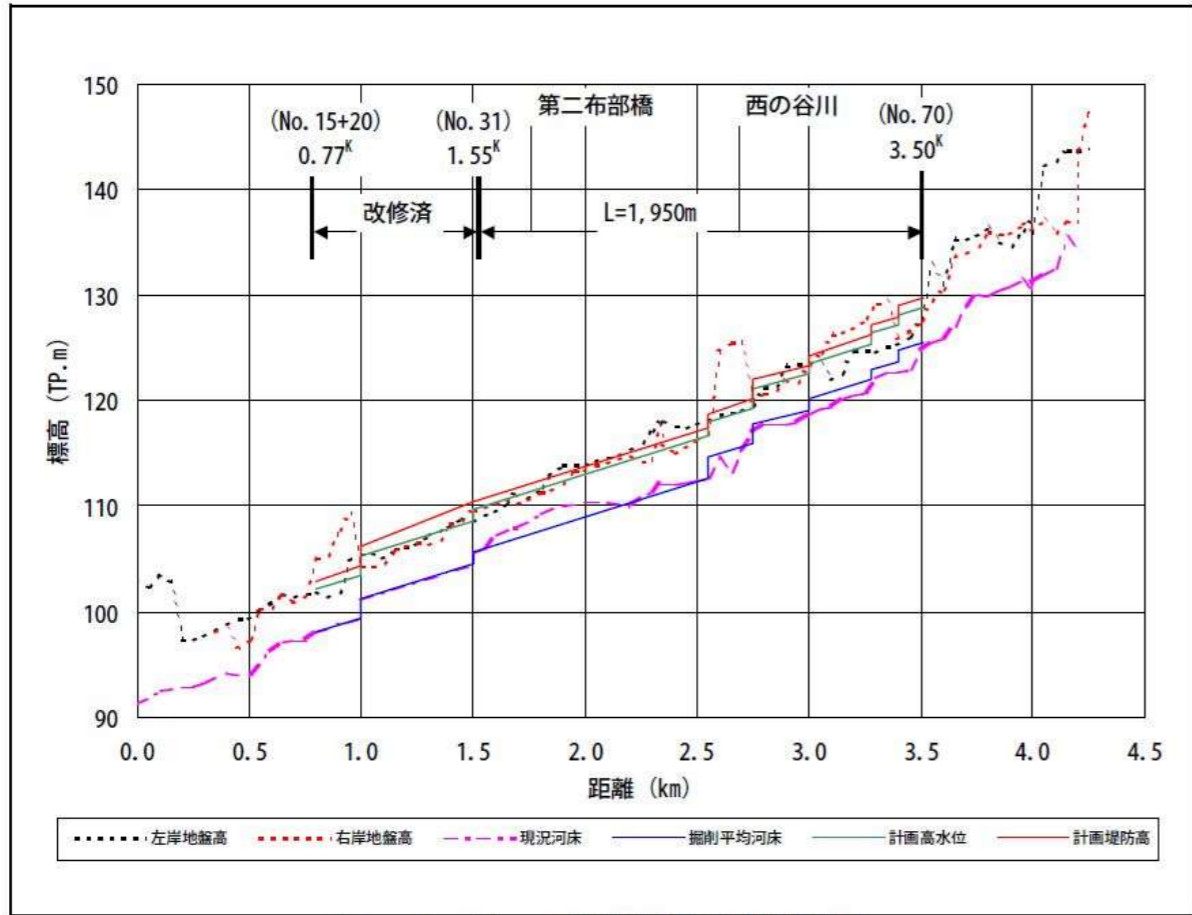
図-3.1.2(6) 飯梨川上流工区縦断面図
