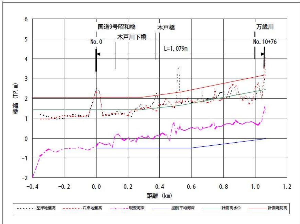
図-3.1.2(14) 木戸川縦断面図
