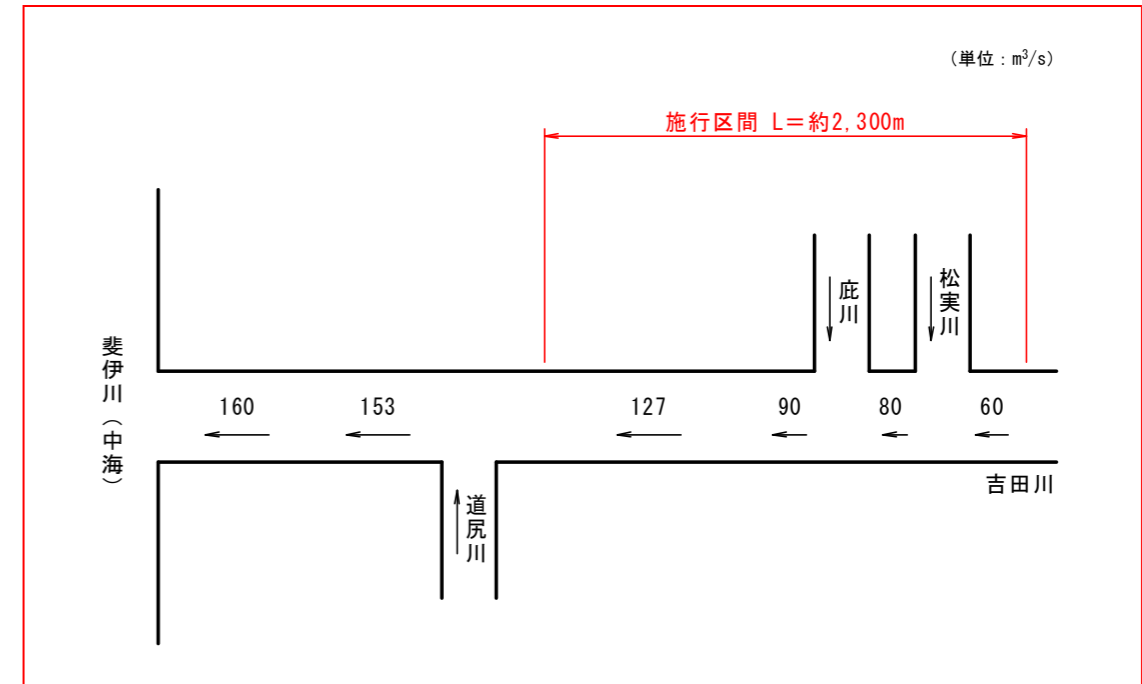
図 4.1-2 吉田川整備計画目標流量図
