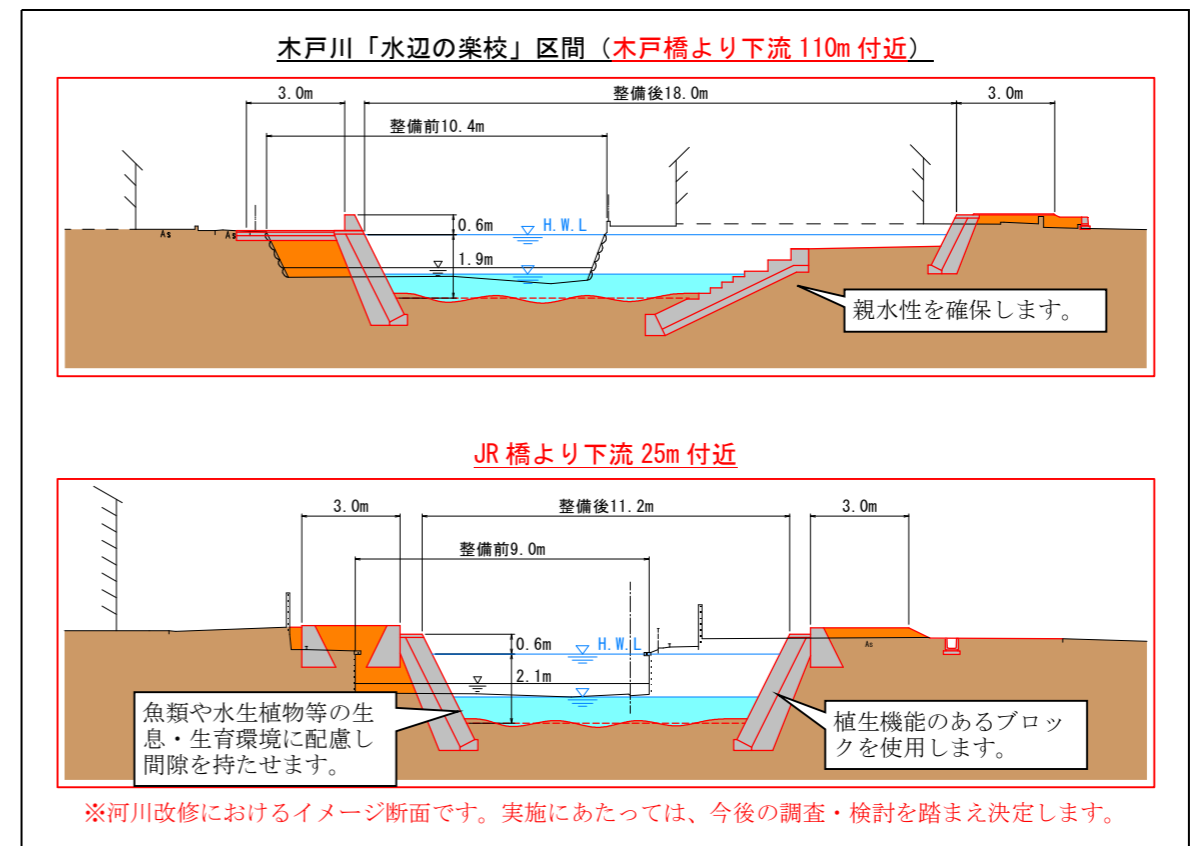
図 4.1-9 木戸川標準横断面図
