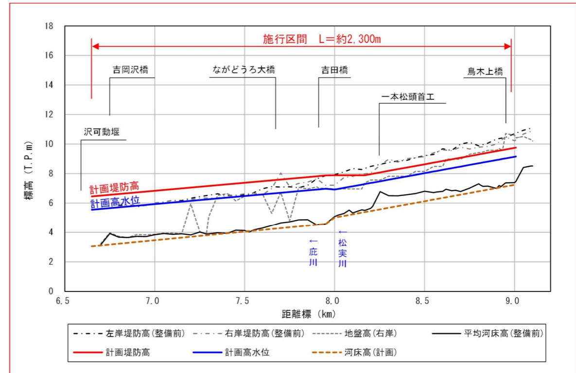
図 4.1-4 吉田川縦断面図
