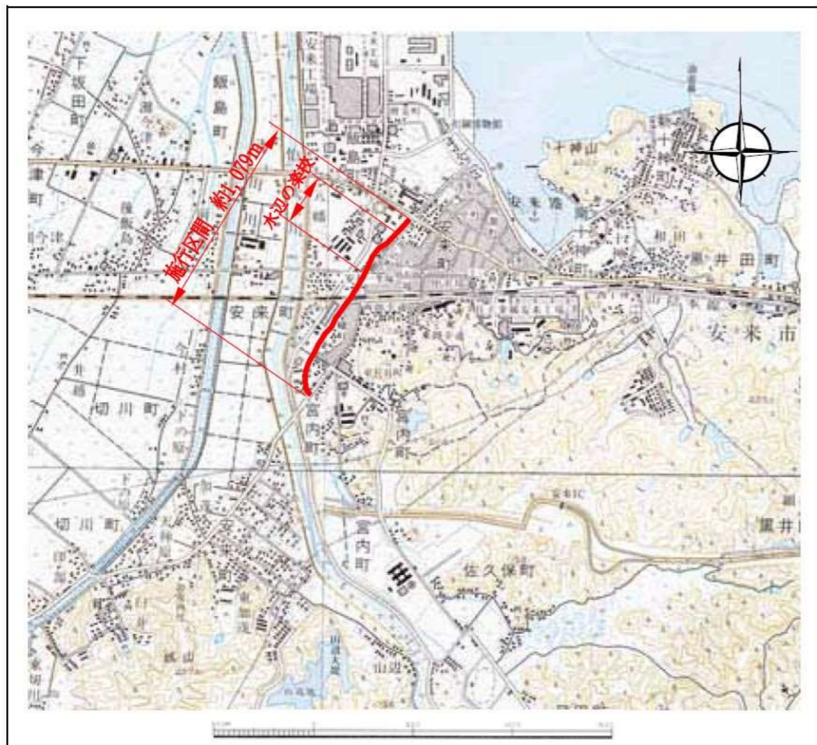
図-3.1.2(13) 木戸川平面図
