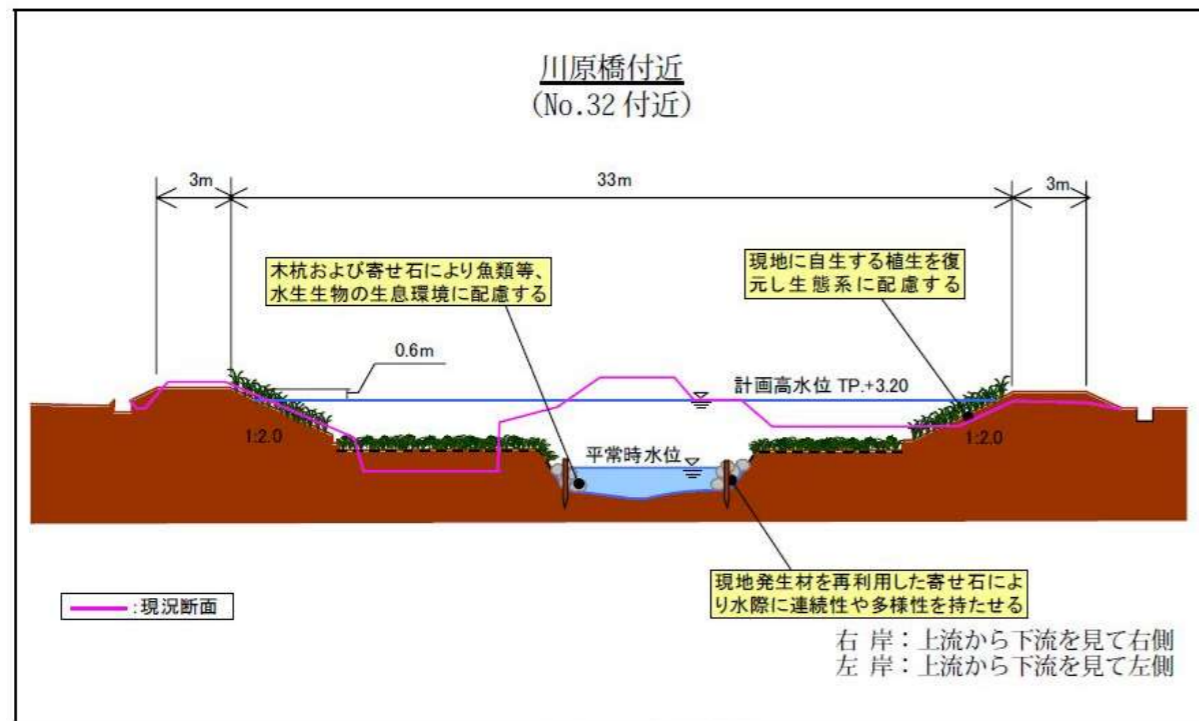
図-3.1.2(19) 標準横断面図
