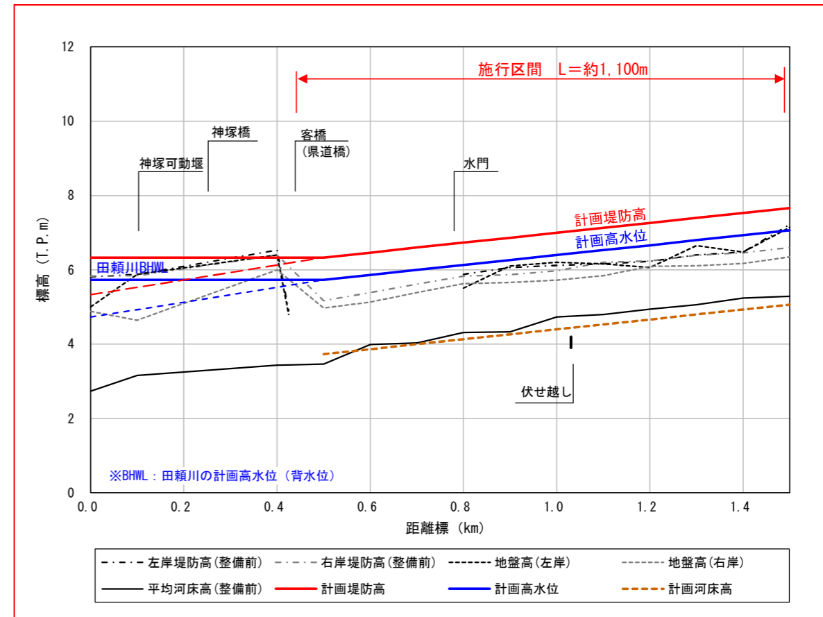
図 4.1-14 津田平川縦断面図
