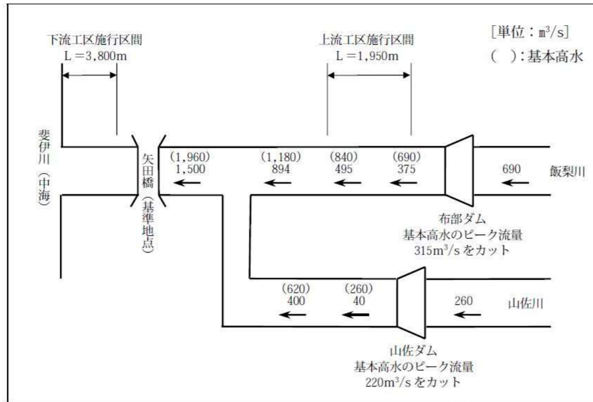
図-3.1.2(1) 飯梨川整備計画目標流量図
