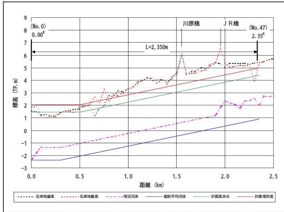
図-3.1.2(18) 田頼川縦断面図
