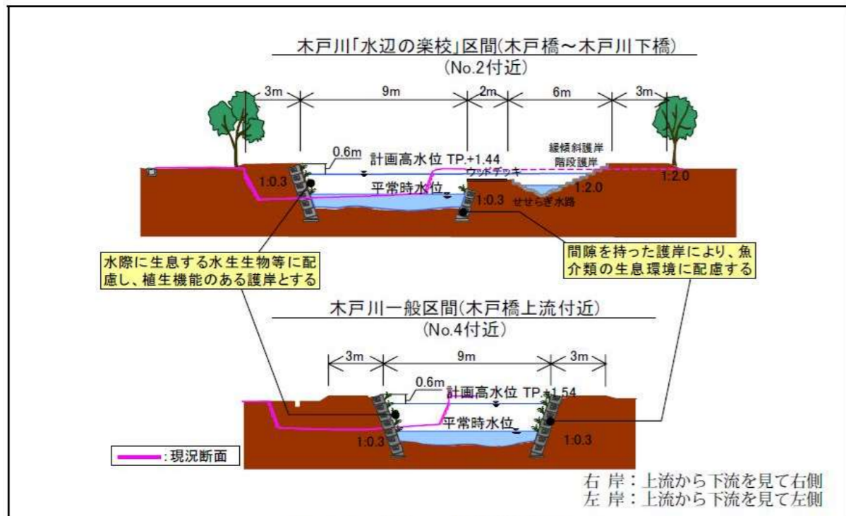
図-3.1.2(15) 標準横断面図
