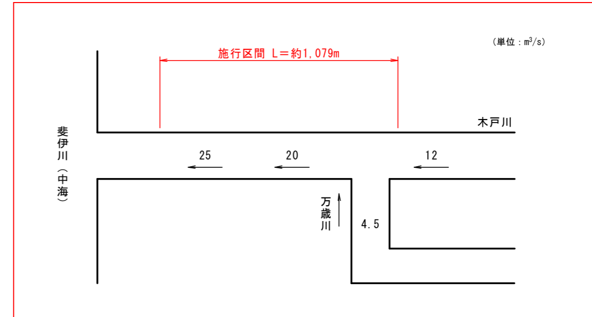
図 4.1-6 木戸川整備計画目標流量図
