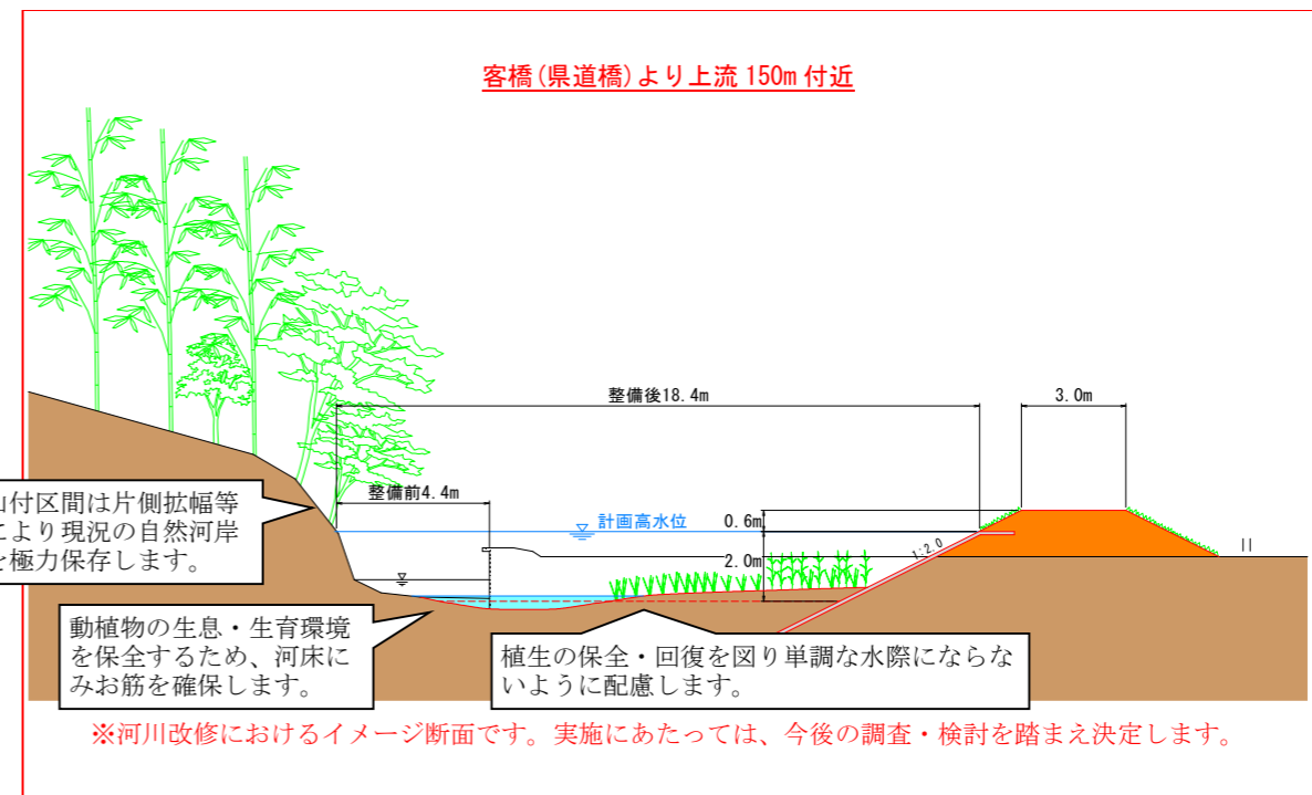
図 4.1-15 津田平川標準横断面図
