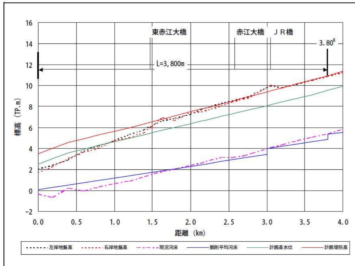
図-3.1.2(3) 飯梨川下流工区縦断面図
