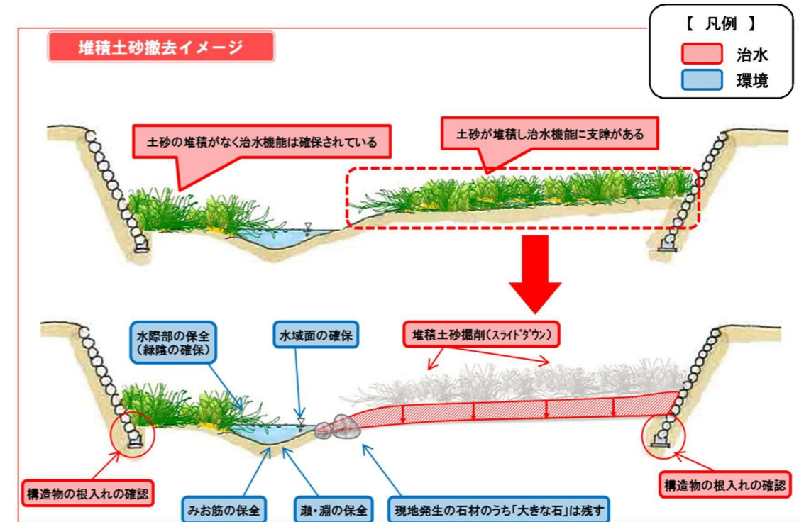
図 4.2-1 堆積土砂撤去イメージ図
