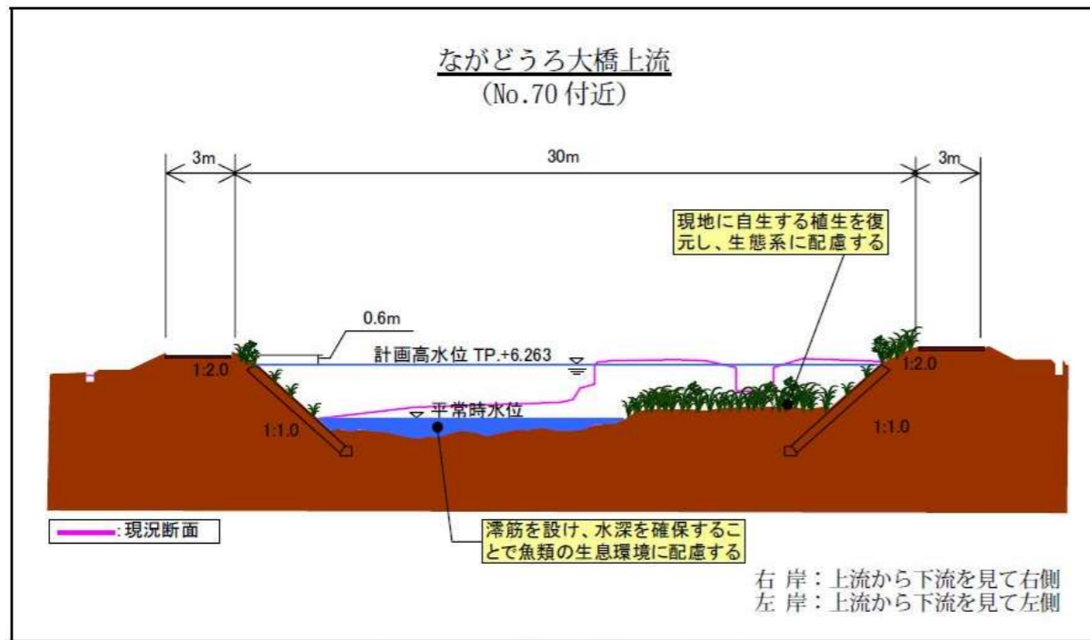
図-3.1.2(11) 標準横断面図
