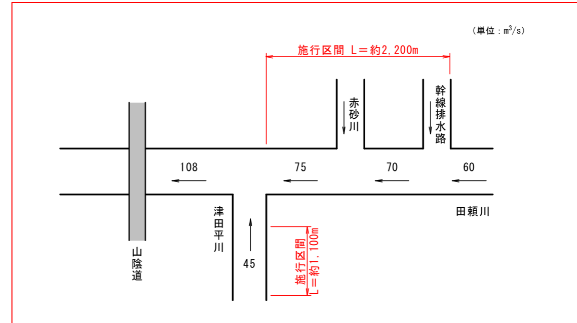
図 4.1-10 田頼川・津田平川整備計画目標流量図
