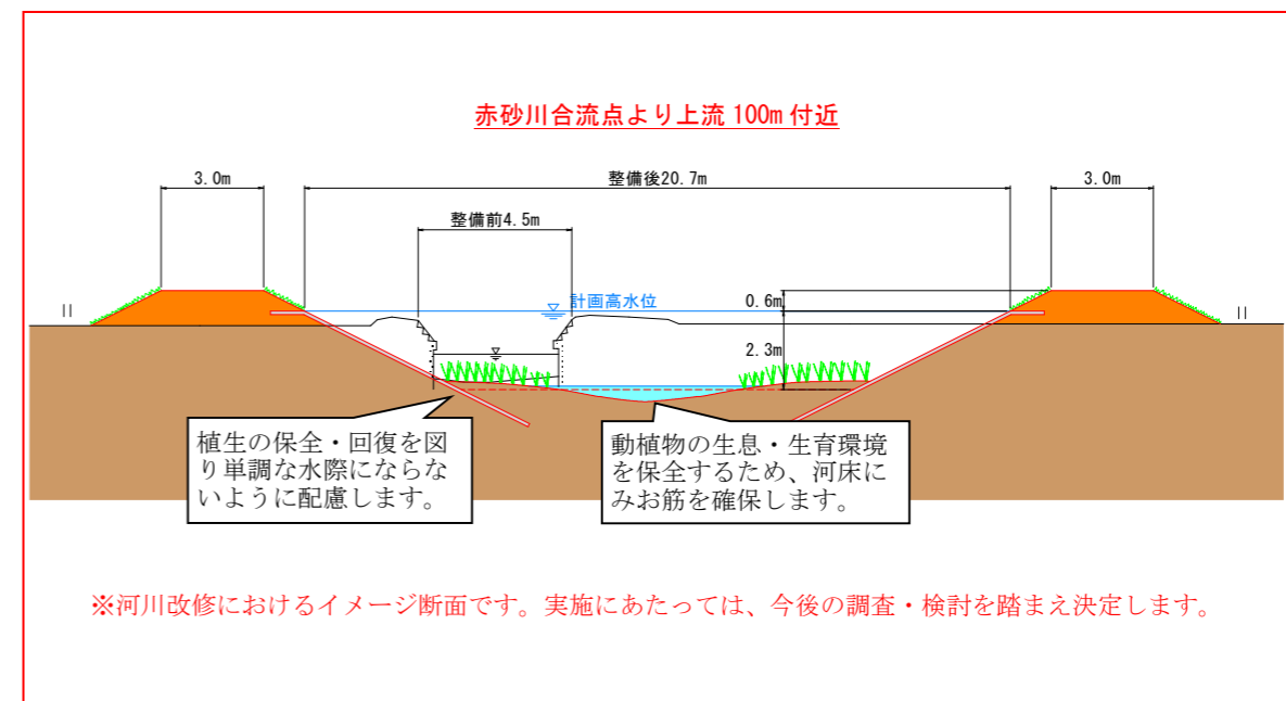
図 4.1-13 田頼川標準横断面図
