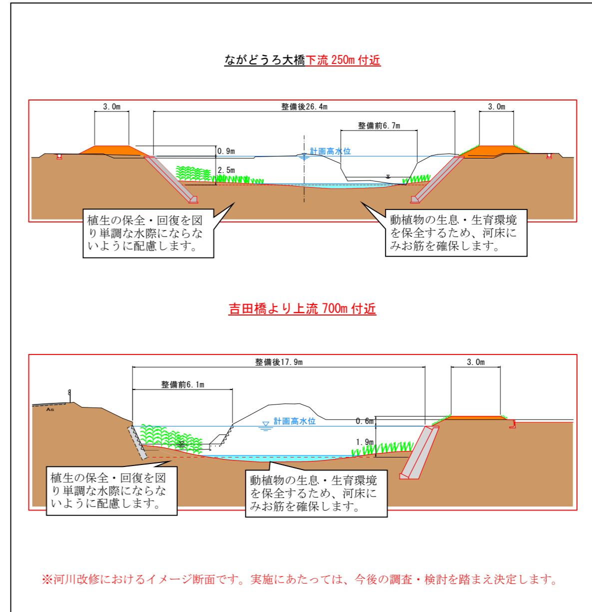
図 4.1-5 吉田川標準横断面図
