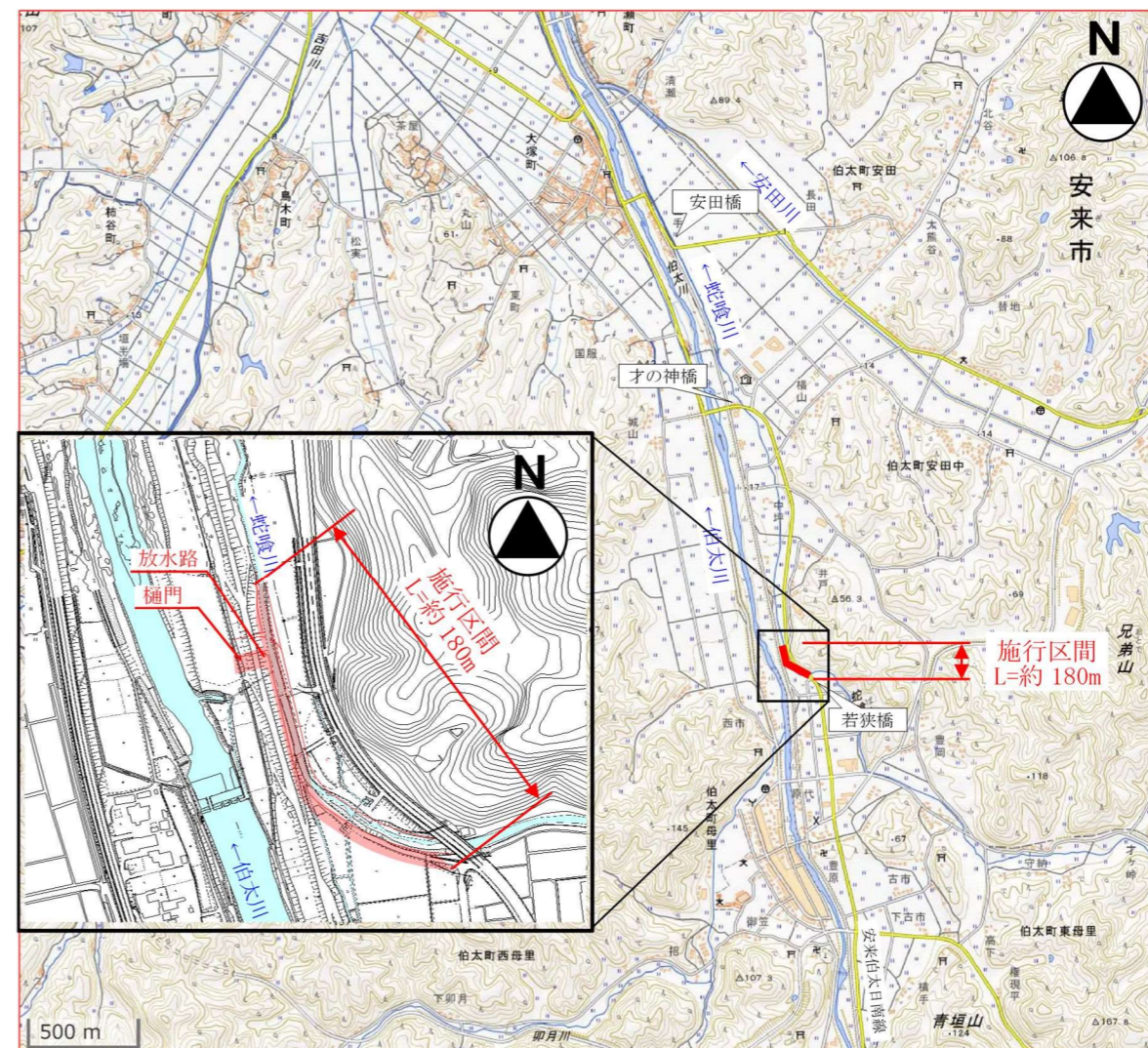
図 4. 1-17 蛇喰川平面図
