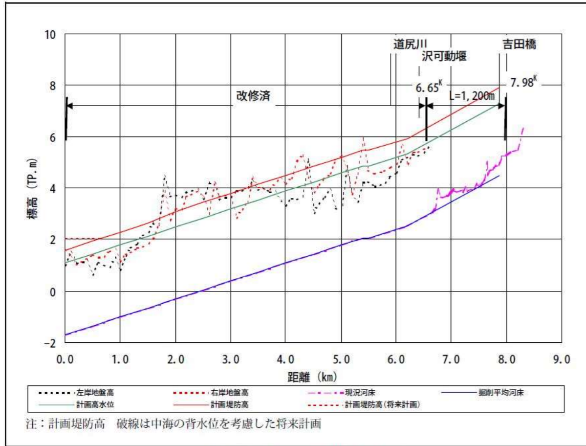
図-3.1.2(10) 吉田川縦断面図
