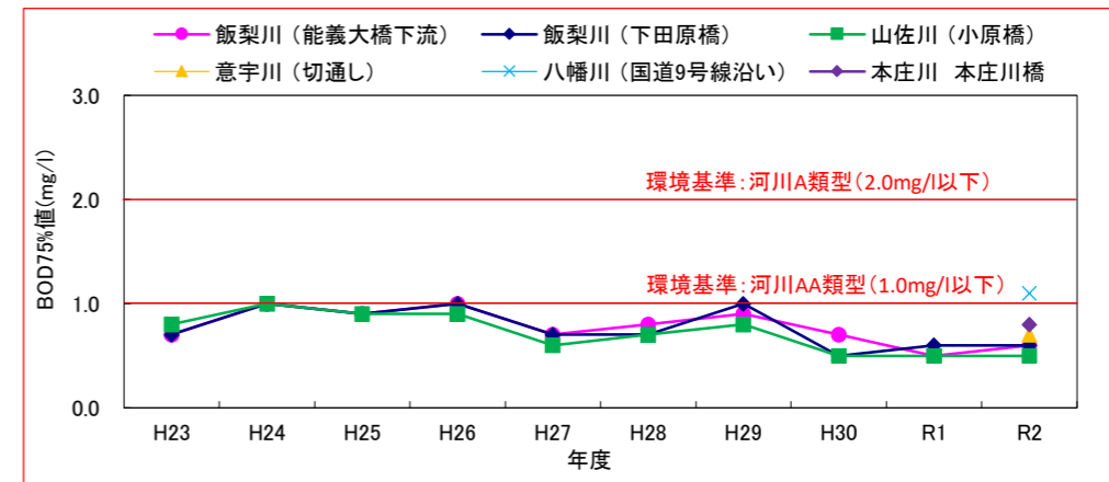
図 3.3-1 BOD75%値 注2) の推移（公共用水域水質測定結果）
