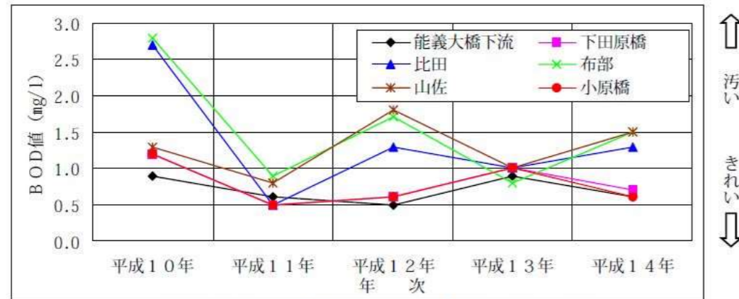
図-1.2.1 飯梨川におけるBOD75%値の推移
