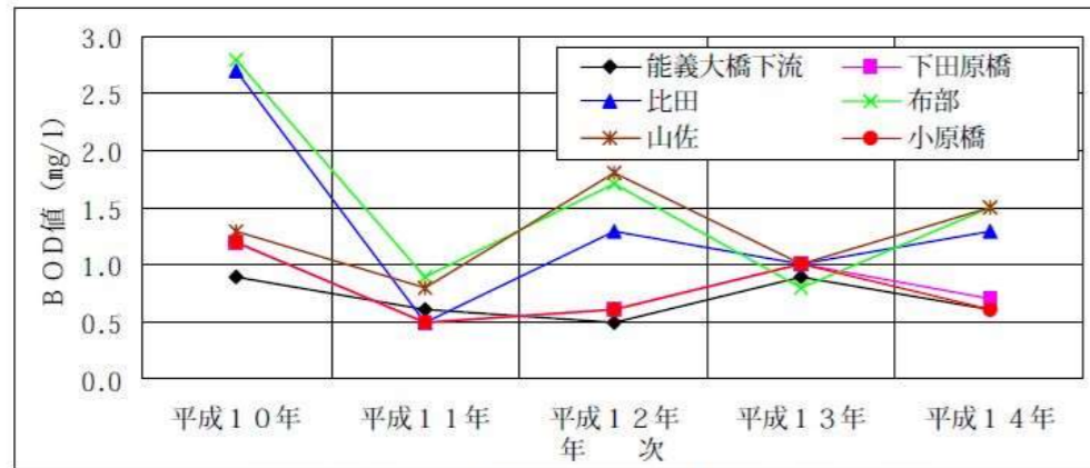
図-1.2.1 飯梨川におけるBOD75%値の推移
