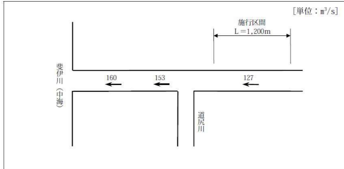
図-3.1.2(8) 吉田川整備計画目標流量図
