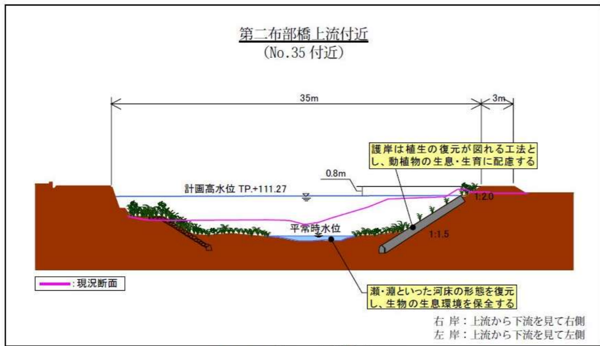
図-3.1.2(7) 標準横断面図
